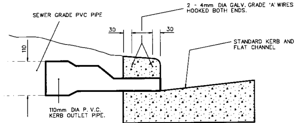
END ELEVATION
